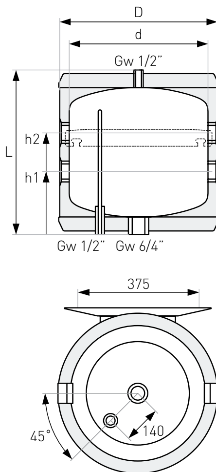
Schéma akumulční nádrže SOLPS 40-140
