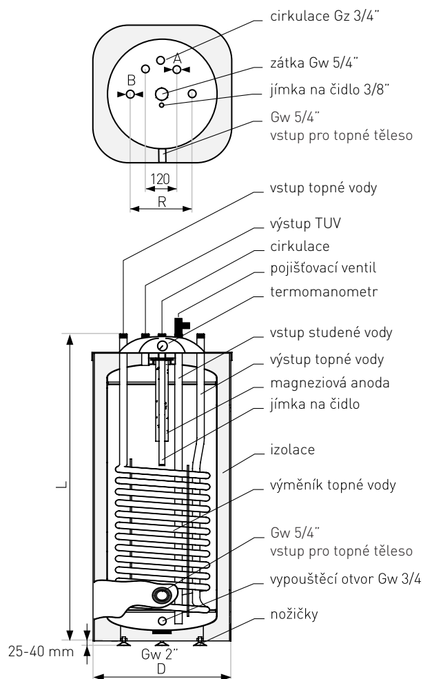
Schéma zásobníku SOLNTR...HV 100 a 120
